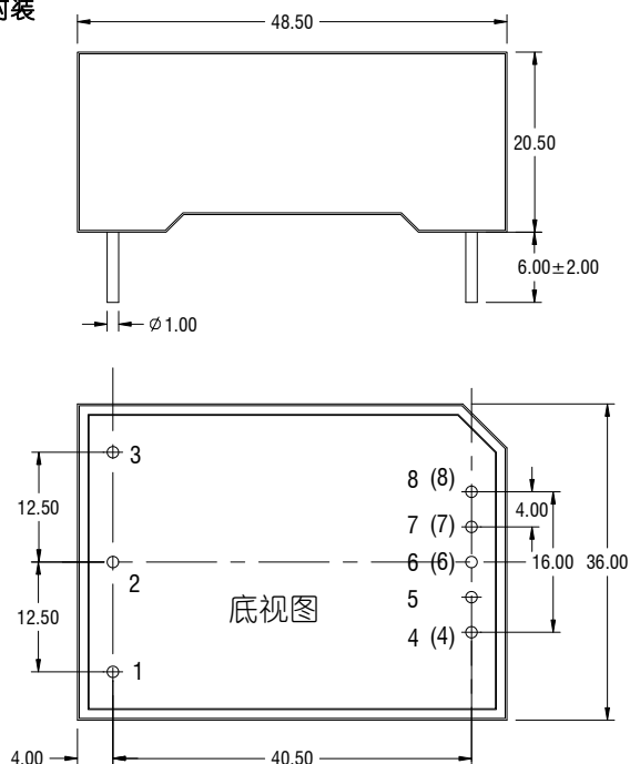
DIP 封装
